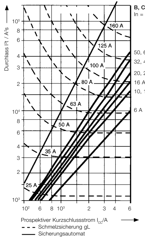
Abb. 2 Durchlassenergie I^2t
